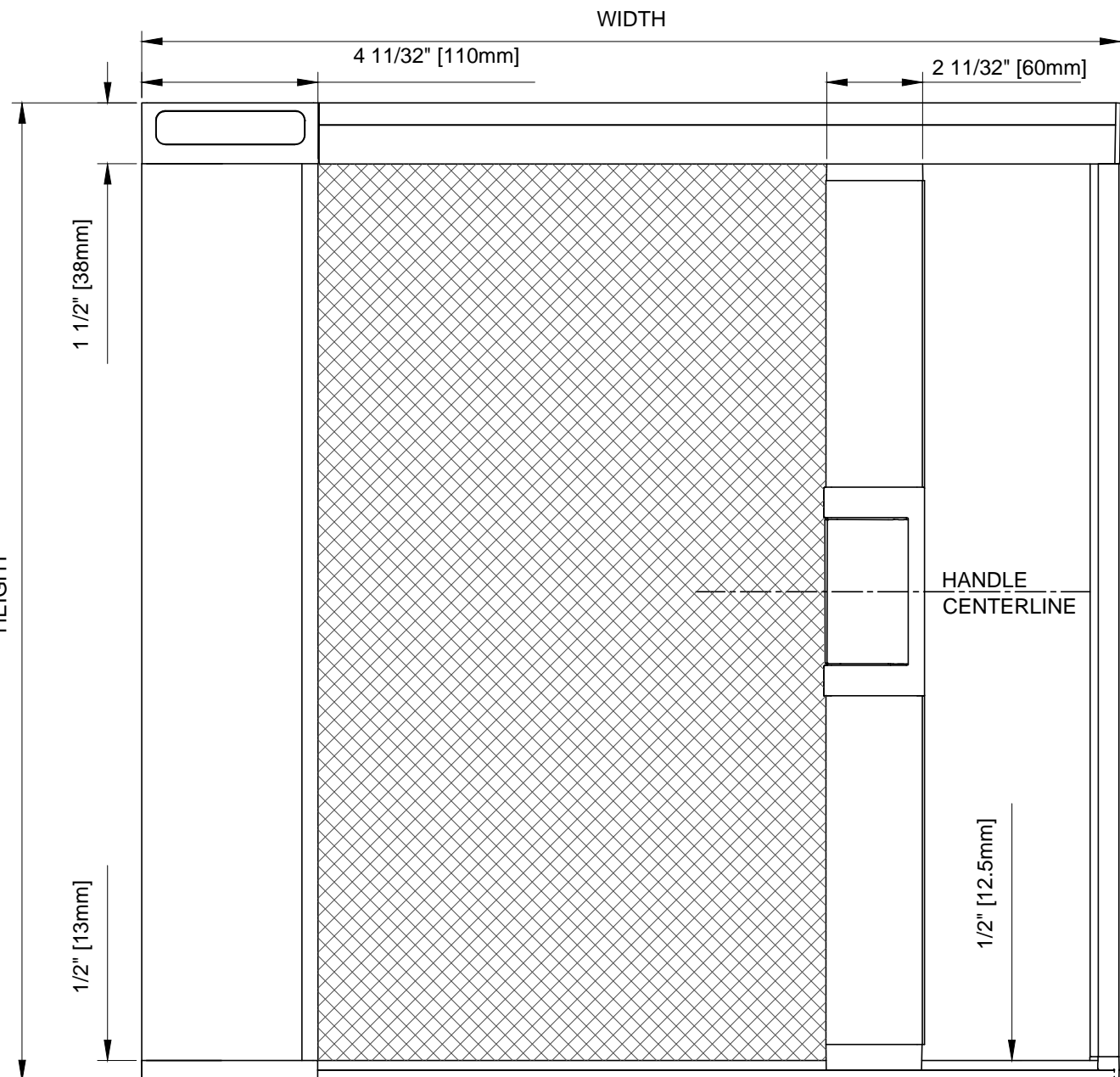
FRONT ELEVATION SCALE: 1:4
